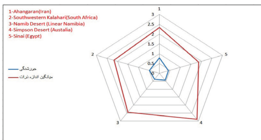
شکل ۹. دیاگرام عنکبوتی مقایسه برآیند میانگین و جورشدهگی تپه‌های ماسه‌ای خطی آهنگران با سایر مناطق دنیا 1) The southwestern Kalarahi (South Africa) (Lancaster, 1986), 2) The Namib Desert linear, Namibia) (Lancaster, 1981), 3) The Simpson Desert (Australia) (Folk, 1971), 4) The Sinai Desert (Egypt) (Tsoar, 1978)
