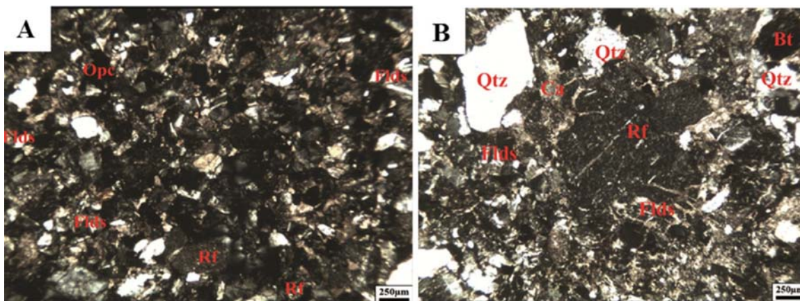
شکل ۴. تصاویر میکروسکوپی ماسه‌سنگ‌ها. (A) آرکوز - آرکوز لیتیک، (B) لیت‌آرنایت فلدسپاردار (نور (Flds)، XPL، فلدسپار، RF: قطعات خرده‌سنگی، Qtz: کوارتز، Ca: کلسیت، Bt: بیوتیت، Opc: کانی اوپک (Kretz, 1983)
