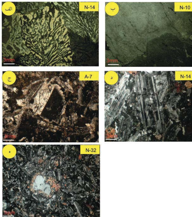
شکل ۲. الف) بافت گرانوفیری در گرانیت‌ها، ب) بافت پرتیتی در فلدسپارها، ج) زونینگ در پلاژیوکلازها، د) پلاژیوکلاز دو نسلی، ه) زونکرست کوارتز با غلاف پیروکسن.
