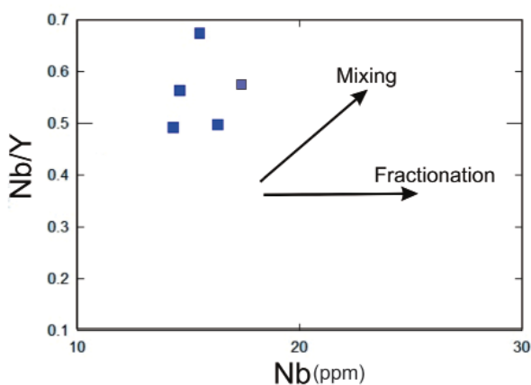
شکل ۸. افزایش میزان Nb در برابر Nb/Y که می‌تواند نشان‌دهنده آلیش ماگمایی در دایک‌ها (الف) و توده نفوذی (ب) باشد (Treuil and Joron, 1975).
