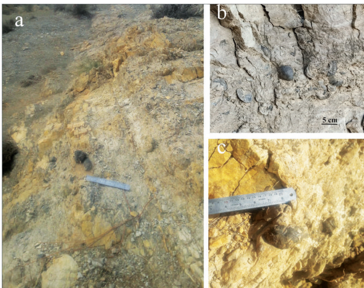
شکل ۶. نمایی نزدیک از واحد سنگ آهک‌های مارنی لوفادار (a) و افق حاوی دوکفه‌ای فراوان (b,c) مربوط به عضو سیمره در برش چینه‌شناسی باغ‌گل
