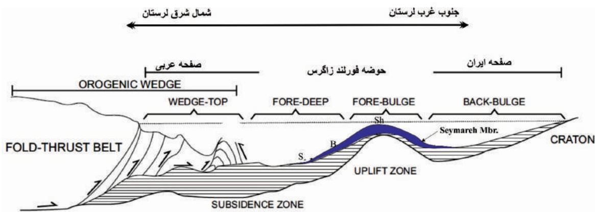
شکل ۱۱. مدل حوضه فورلند زاگرس و تغییرات ضخامت و محدوده گسترش عضو سیمره در برش‌های شیخ‌مکان (Sh)، باغ‌گل (B) و سیاه‌دره (S) برگرفته از DeCells and Giles, 1996 با تغییرات
