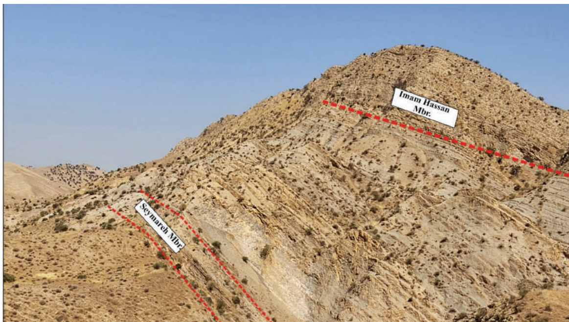
شکل ۵. نمایی کلی از سازند گورپی و بخش‌های مختلف آن به‌ویژه عضو سیمره در برش چینه‌شناسی باغ‌گل، تاکدیس سلطان
