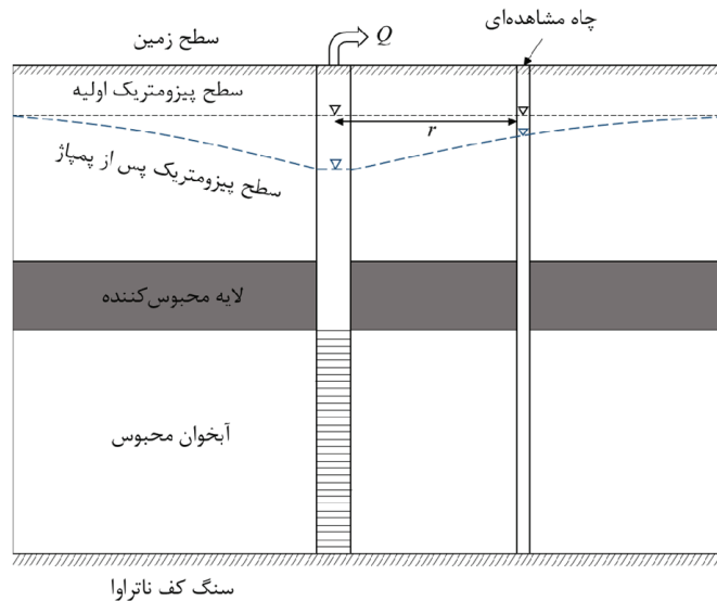
شکل ۱. نمای شماتیکی آبخوان محبوس به همراه چاه پمپاژ با نفوذ کامل
