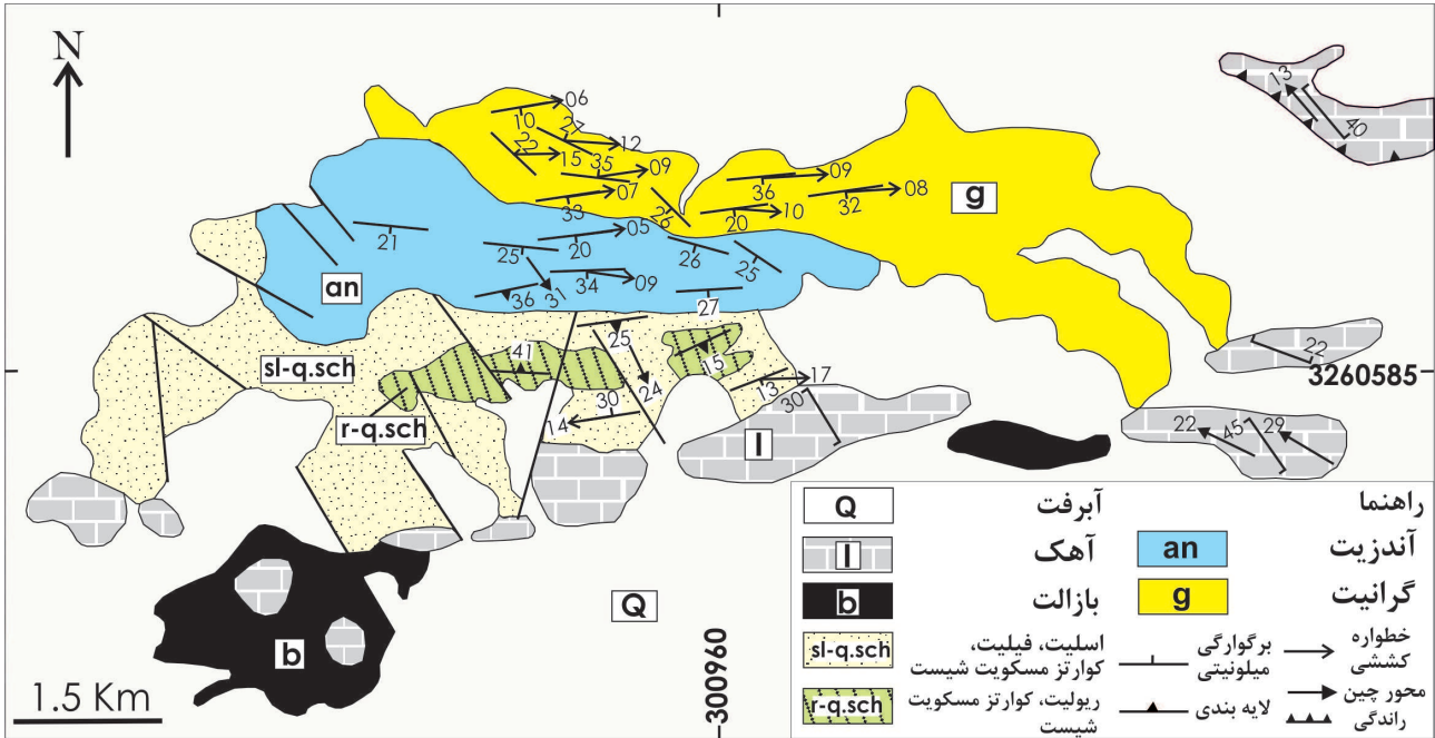
شکل ۸. نقشه زمین شناسی ناحیه دوچاه‌زها که بر پایه تصاویر ماهواره‌ای ترسیم شده است (اندازه‌گیری‌های ساختاری روی آن پیاده شده است).
