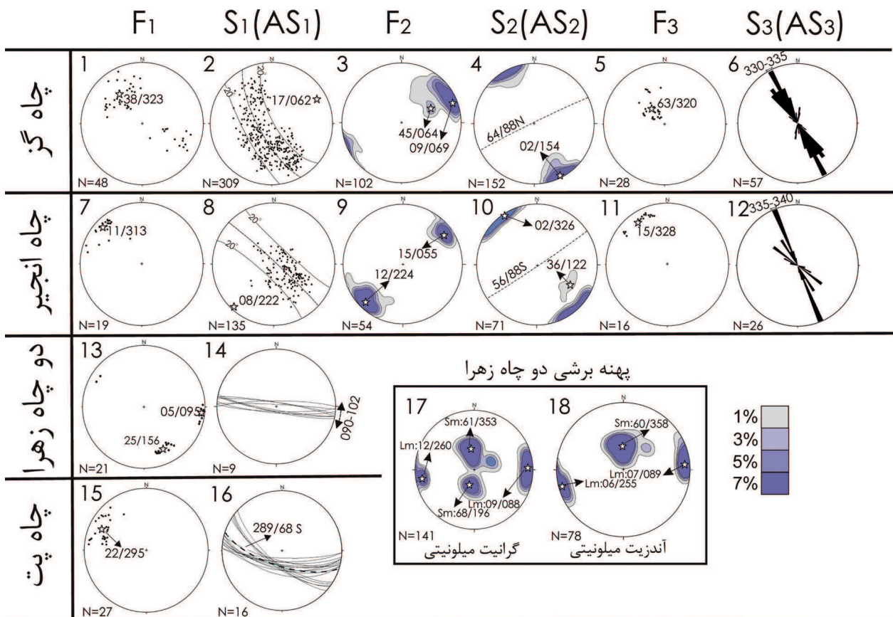
شکل ۶. استریوت‌های عناصر ساختاری مناطق چاه‌گز، چاه‌انجیر، دوچاه‌زهرا و چاه‌پت. داده‌ها در نیمکره پائینی و بر روی شبکه هم مساحت تصویر گردیده‌اند و در شکل‌های ۱۷، ۱۸ و ۵، ۳، ۹، ۴، ۱۰، ۱۱ و ۱۲ بر اساس ۵، ۳، ۱ و ۷٪ توزیع داده‌ها در ۱٪ مساحت کنتوربندی شده‌اند. ستاره‌ها موقعیت میانگین داده‌های ساختاری را نشان می‌دهند.
