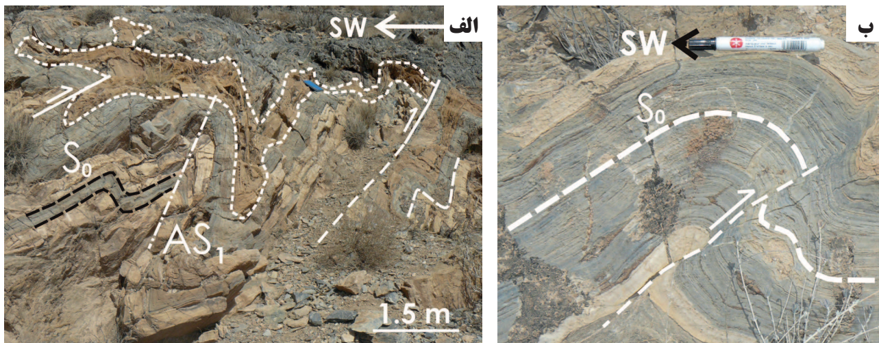
شکل ۹. چین‌های گامه اول در واحد مرمری شمال چاه‌پت. الف) برای جبران فضای حاصل از جریان‌یافتگی واحد نامقاوم قهوه‌ای رنگ (مشخص شده با خط چین)، راندگی‌هایی در واحدهای مقاوم توسعه یافته‌اند، ب) راندگی هم‌زمان با چین‌خوردگی عمل نموده و توسعه آن در داخل چین متوقف شده است.
