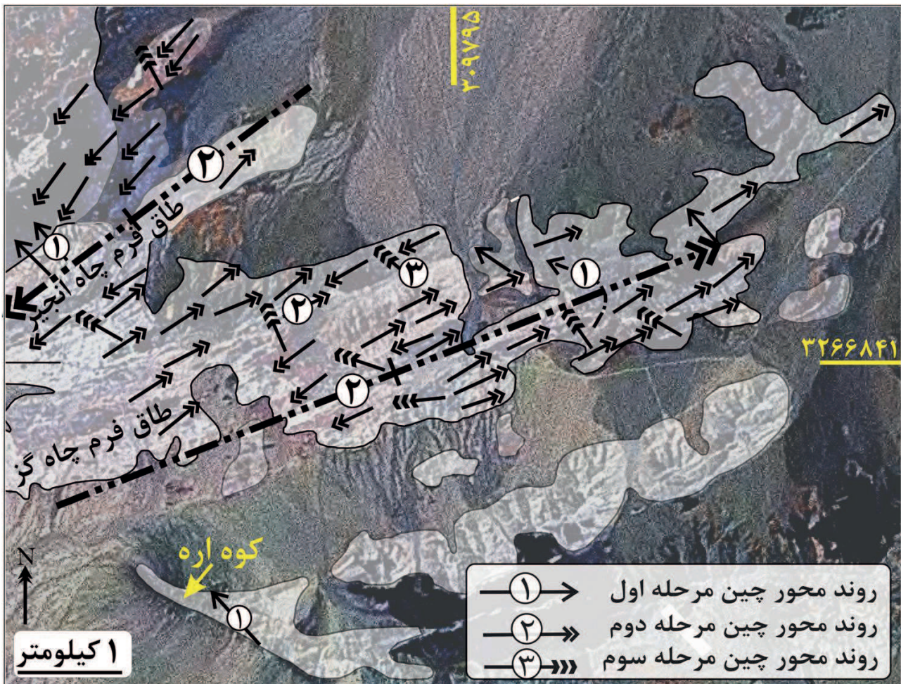
شکل ۳. تصویر ماهواره‌ای و نقشه ساده شده ساختاری از موقعیت طاق فرم‌های با مقیاس کیلومتری گامه دوم و روند محوری چین‌های متوسط مقیاس هر سه گامه دگرریختی در ناحیه چاه‌گز و چاه‌انجیر.
