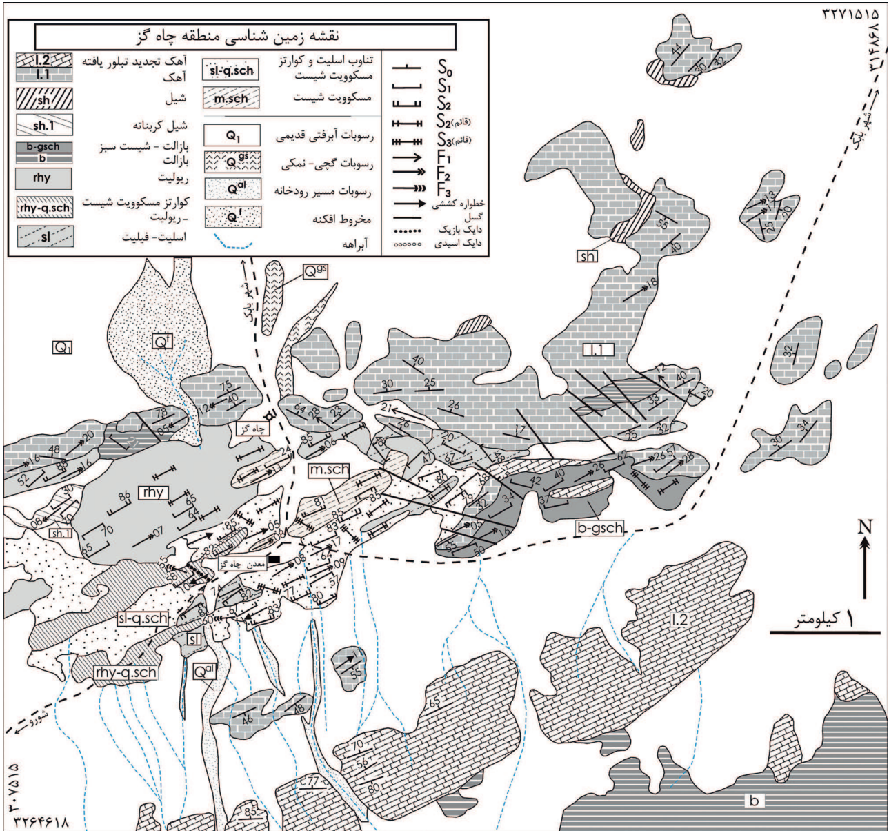
شکل ۴. نقشه زمین شناسی ساختاری ناحیه چاه گز.
