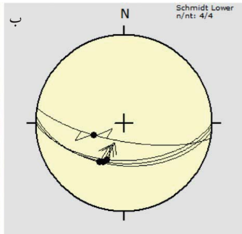
شکل ۶. الف) نحوه عمل کرد گسل RF3 در منطقه، (Db عضو دولومیتی سازند بهرام، Dsh1 شیشتو ۱ می باشد)، ب. آثار لغزش روی سطح گسل (زاویه ریک حدود ۷۵ درجه) و تصویر استریو گرافیک گسل RF3 با جهت لغزش این گسل.
