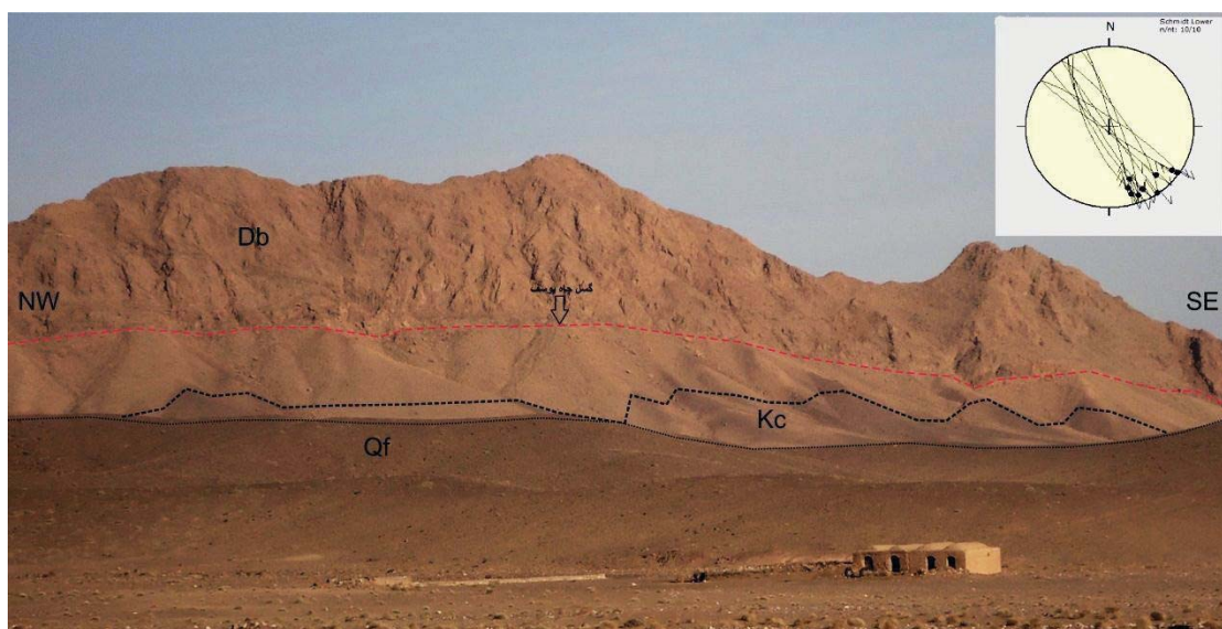
شکل ۵. نمایی از گسل امتدادلغز چاه یوسف به همراه استریونت صفحات گسلی برداشت شده. Db عضو دولومیتی سازند بهرام، Kc کنگلومرای کرتاسه و Qf مخروط افکنه‌های کوتاه‌تر.
