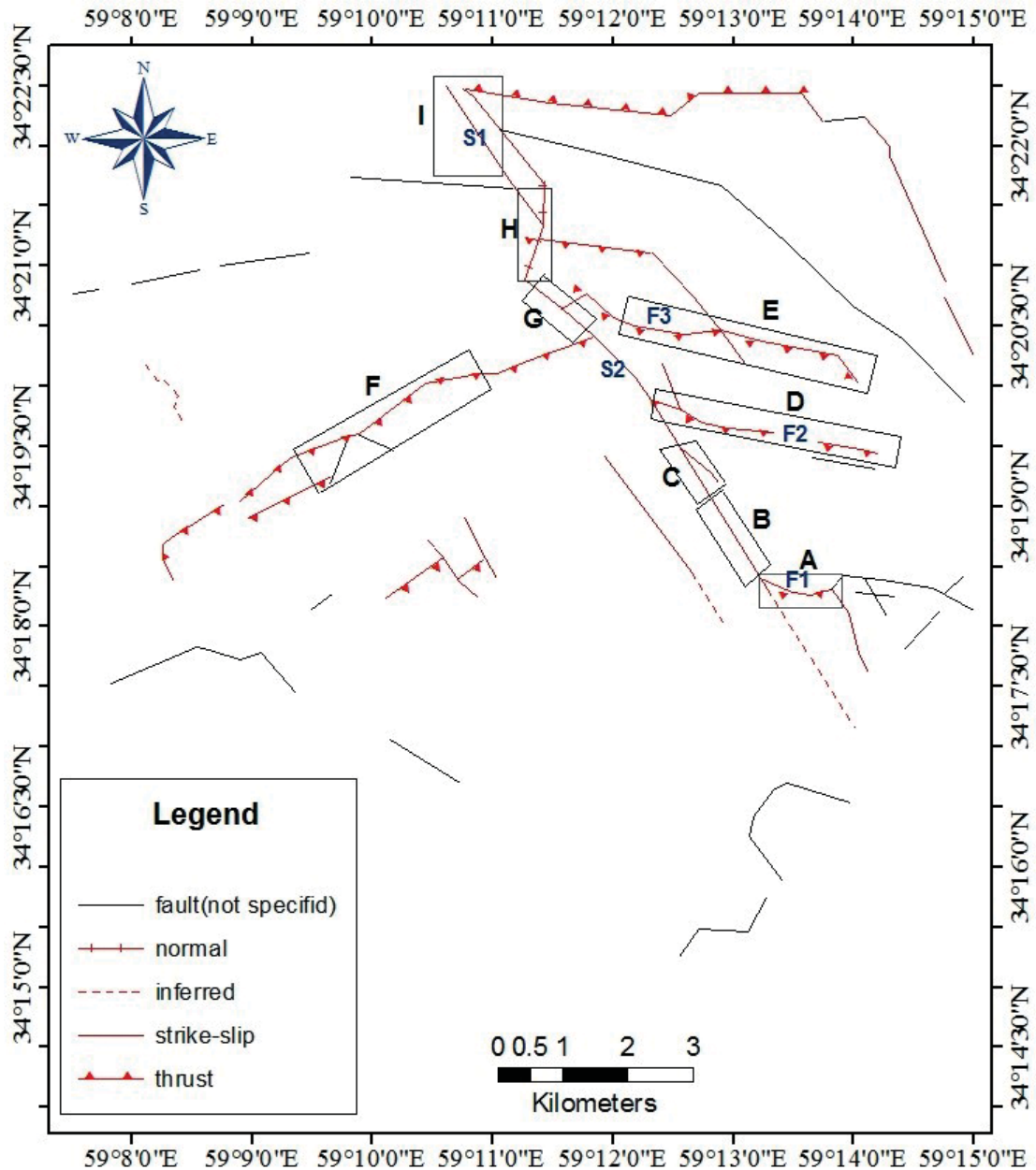
شکل ۴. نقشه ساختاری منطقه مور مطالعه. (ایستگاه‌ها با کادرهای مشکی مشخص شده‌اند).
