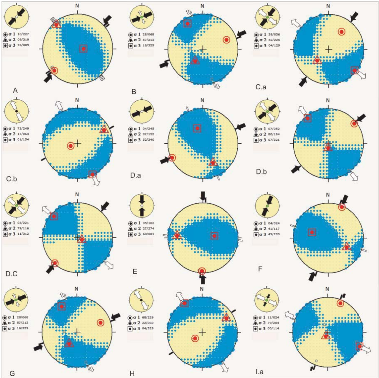
شکل ۱۱. نتایج تنش برگشتی در ایستگاه‌های مختلف. موقعیت \sigma_1 ، \sigma_2 و \sigma_3 در هر استریو پلات به ترتیب با \odot ، \triangle و \square مشخص شده است و جهت نهایی کشش یا فشارش با پیکان‌های توپر نشان داده شده است. ایستگاه‌های I.a و B، C.a، D.b، D.c، G رژیم زمین‌ساختی راست‌الغز (امتدادلغز محض یا امتدادلغز کششی)، ایستگاه‌های A، D.a، E، F رژیم زمین‌ساختی فشارشی و دو ایستگاه C.b و H حاکی از وجود رژیم زمین‌ساختی کششی می‌باشند.
